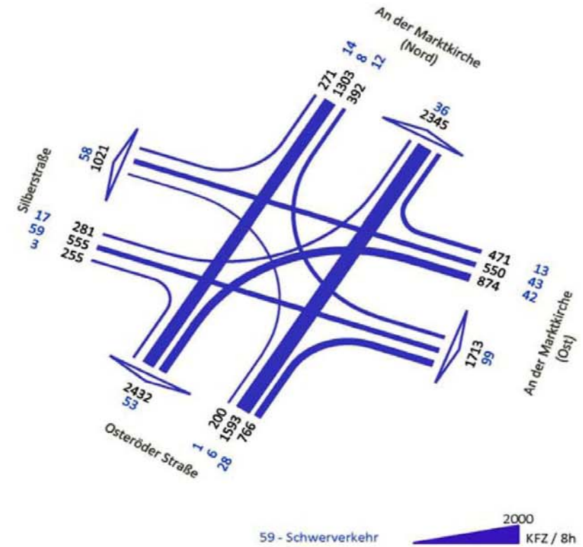
Zählergebnisse [Kfz/8 Std.]
