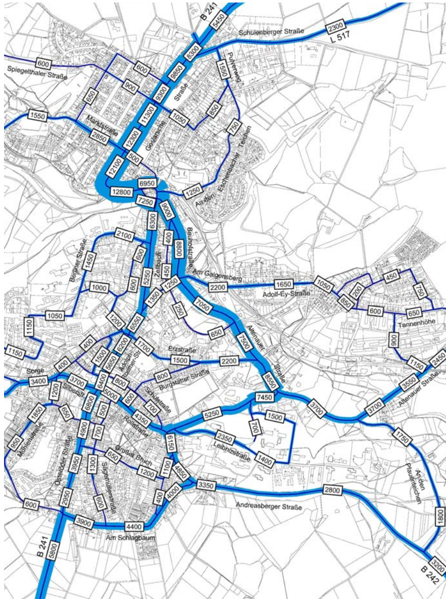
Prognosebelastungen 2030 im Planfall
