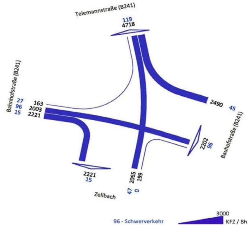
Zählergebnisse [Kfz/8 Std.]
